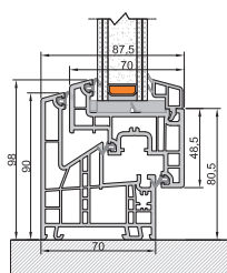
Nodo Inferiore Telaio L
