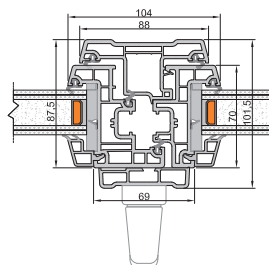
Nodo Centrale Sistema 70 EVO DESIGN
