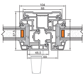
Nodo Centrale Sistema 70 EVO
