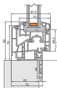
Nodo Inferiore Telaio Z40
