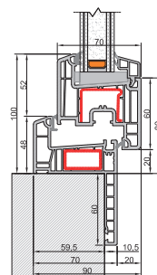
Nodo Inferiore Anta squadrata telaio Z60
