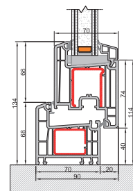
Nodo Inferiore Anta maggiorata telaio L
