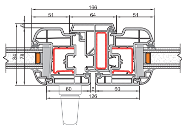
Nodo Centrale Anta arrotondata
