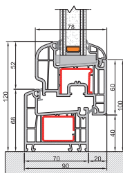
Nodo Inferiore Anta arrotondata telaio L
